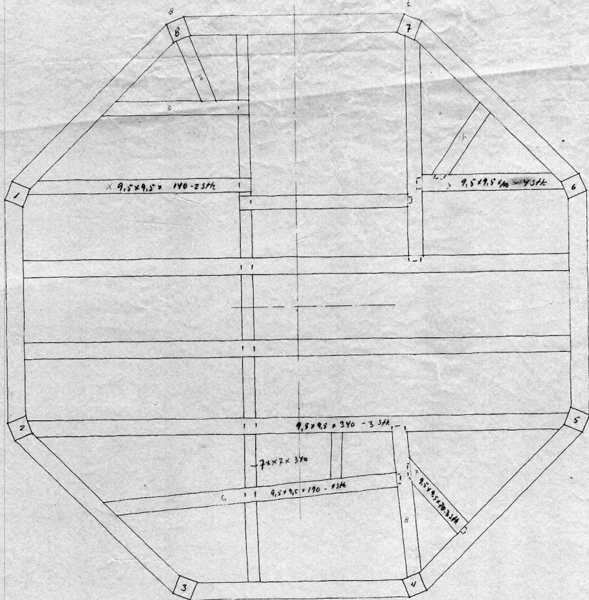
Bjælkelag i broloft, mål 1:25
