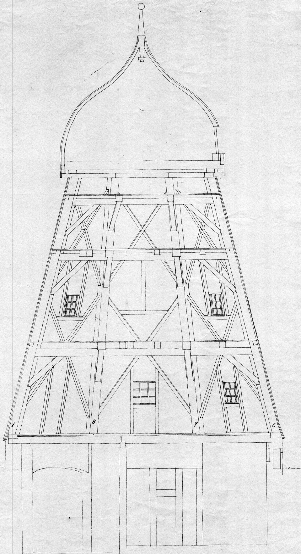
Snit A-A, målt 1:25 A 106 C 090
